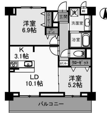
B`type 59.88㎡ 2LDK
